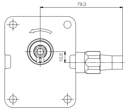
Bomba giro izquierda Counterclockwise rotation pump
