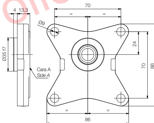
Tapa tipo 27 / Front flange type 27
